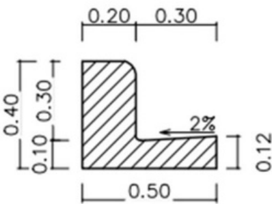
Tipo 2: Contén con una altura de 0.40 m y una base de 0.50 m.
