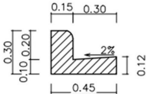
Tipo 1: Contén con una altura de 0.30 m y una base de 0.45 m.
